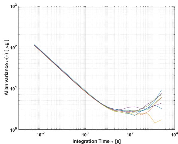
图 12: 艾伦方差
