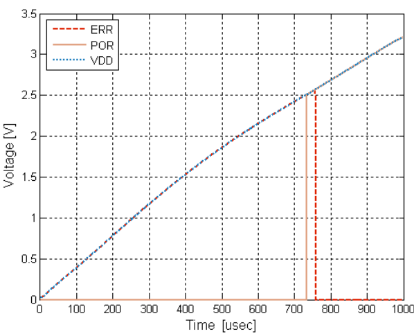
图 39：使用推荐电路时典型的传感器上电序列
