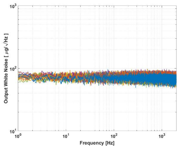
图 23: 典型白噪音
