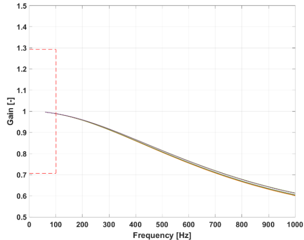
图 16: 频率响应
