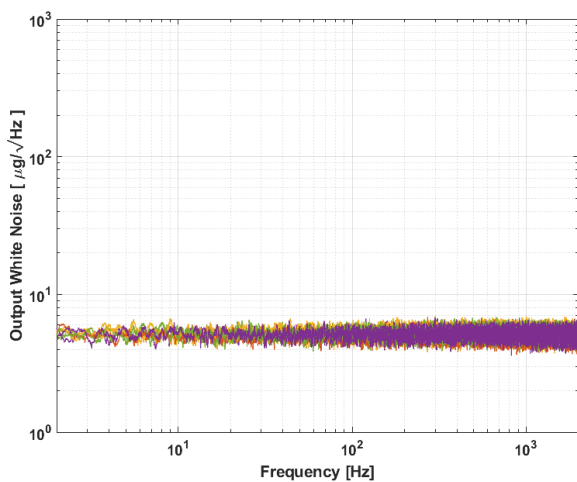
图 5: 典型白噪声
