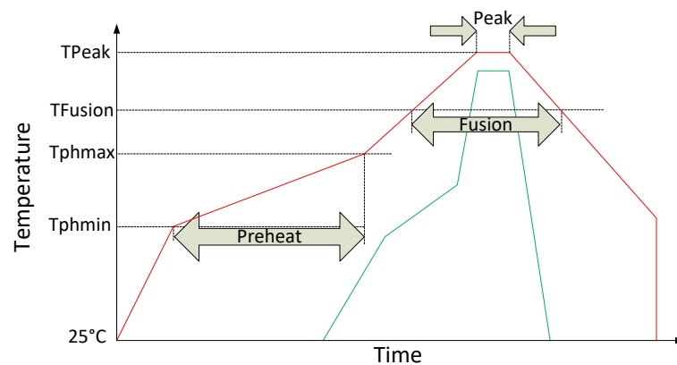
图 46: 焊接温度曲线
