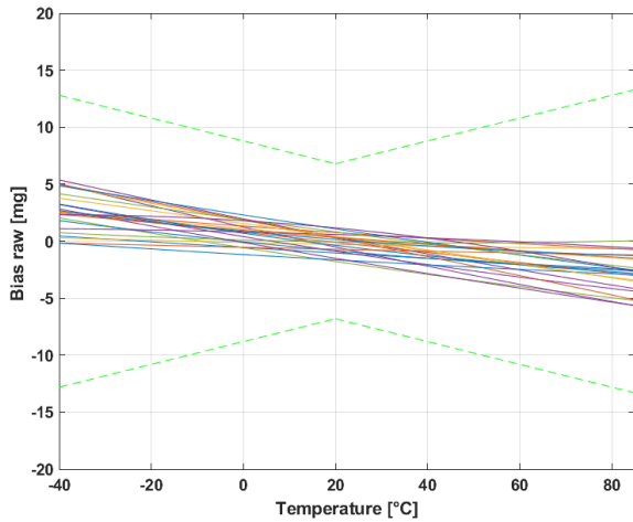
图 1: 原始零偏
