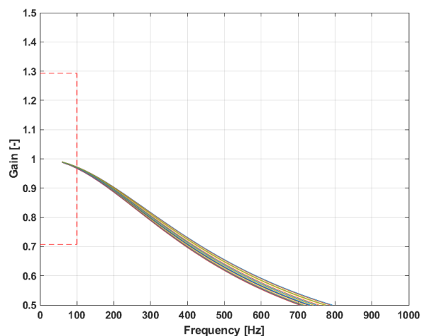
图 10 : 频率响应
