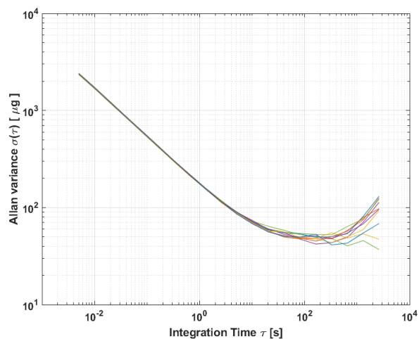
图 36: 艾伦方差
