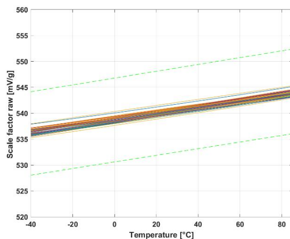
图 8: 原始比例因子
