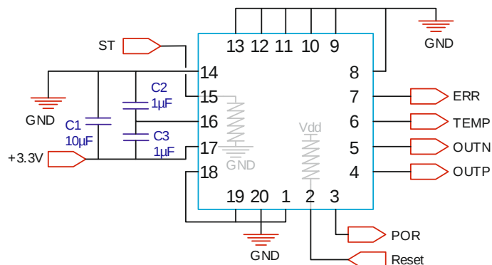
图 38：邻近电路&内部上拉/下拉(pull-up/down)
