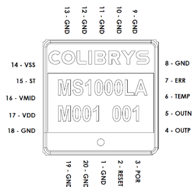
图 37：引脚俯视图
