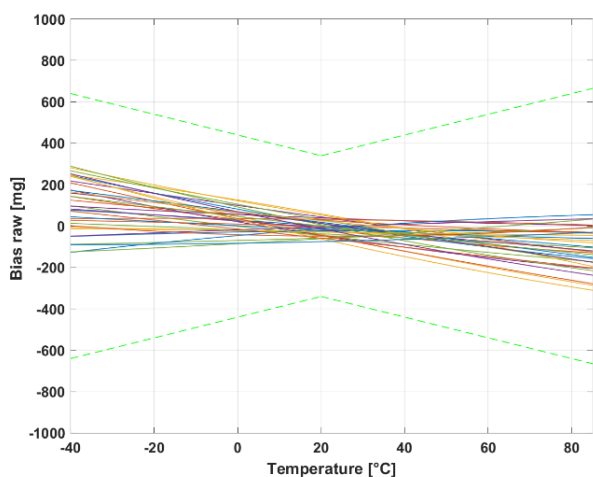
图 31: 原始零偏
