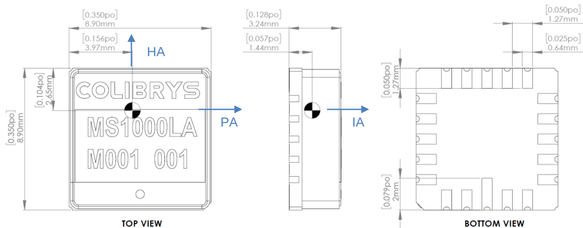
图 43 : 包装外观尺寸, 单位是 mm [inch]
