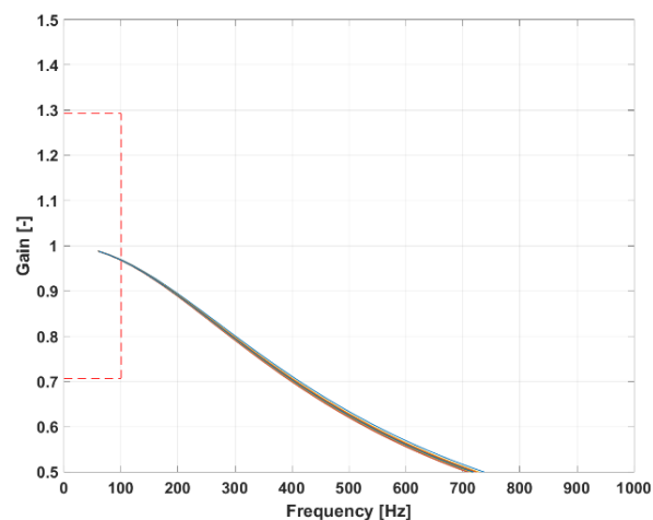
图 34 : 频率响应
