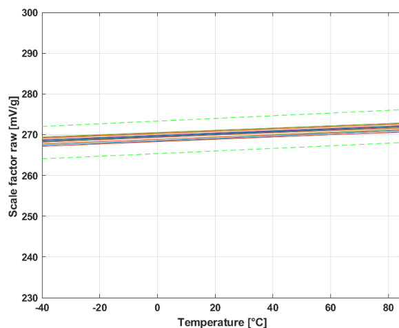
图 14: 原始比例因子
