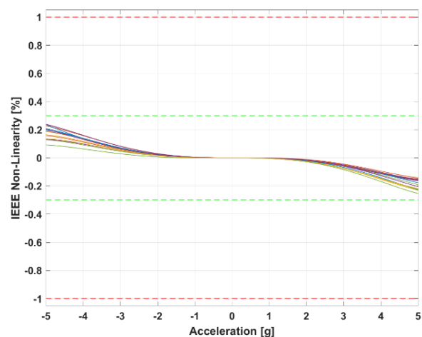
图 9 : 非线性度 IEEE
