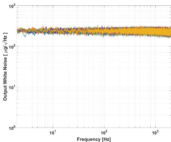
图 35: 典型白噪音
