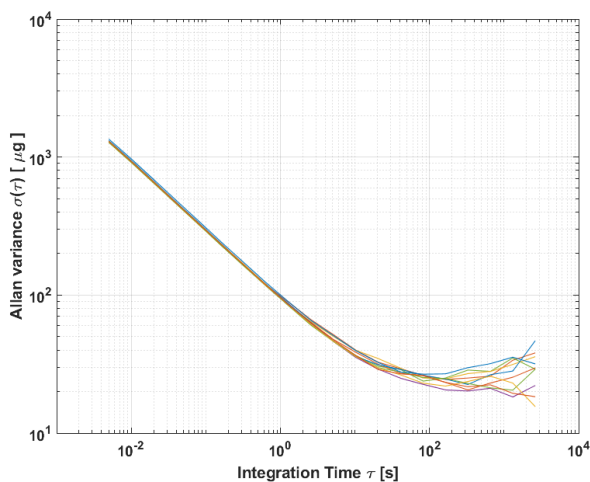
图 30: 艾伦方差
